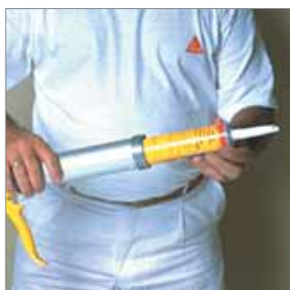
Introducción del cartucho en la pistola.
